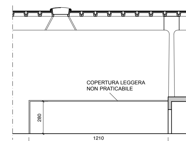
SEZIONE A-A su sala mostra
