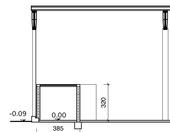
SEZIONE B-B su magazzino
