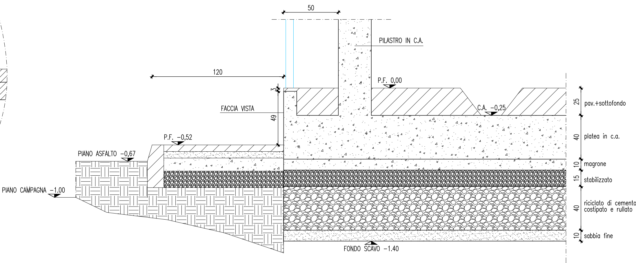
PARTICOLARE STRATIGRAFIA DI FONDAZIONE E MARCIAPIEDI 1:20
